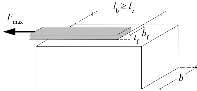
Figura 7-5 – Forza massima trasmissibile da un rinforzo con FRP.
